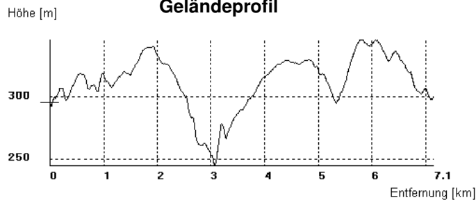
Geländeprofil
